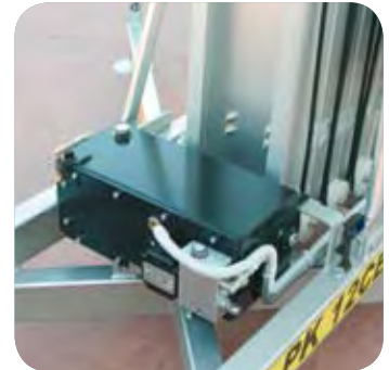
Centraline a 220 Volt con motore immerso nell'olio. 220 Volt gearcase with motor dipped in oil.
